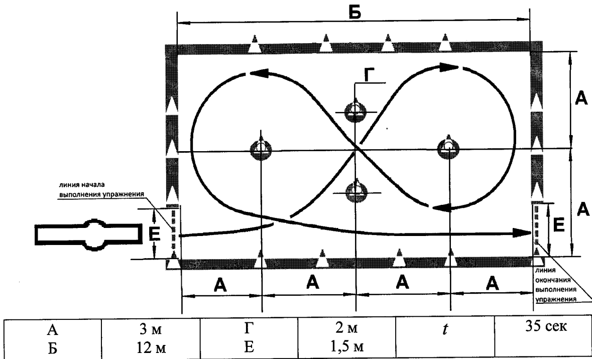
Рисунок 1. Схема и размеры элемента упражнения № 1 – Габаритная восьмерка»
